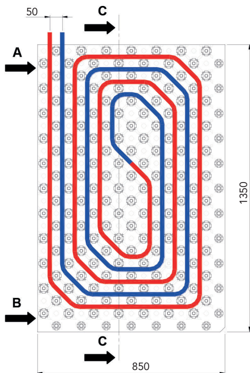
Figure 1 – Exemple de développement du tuyau et principales dimensions*
